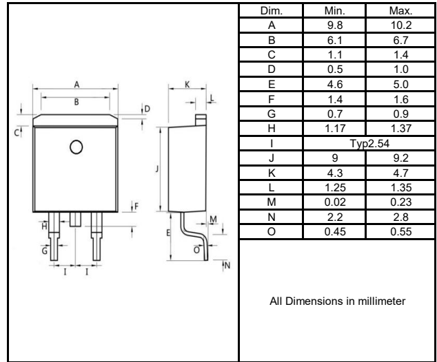
TO-263C
