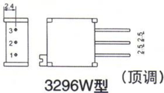
共有尺寸图
