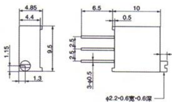
共有尺寸图
