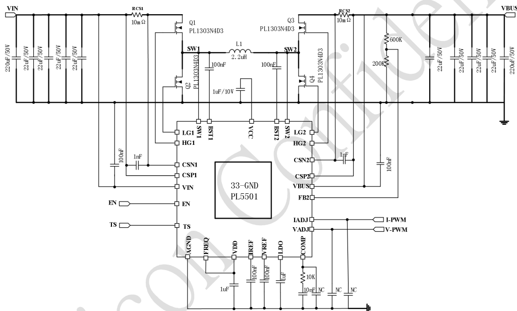
Fig. 31 Schematic
