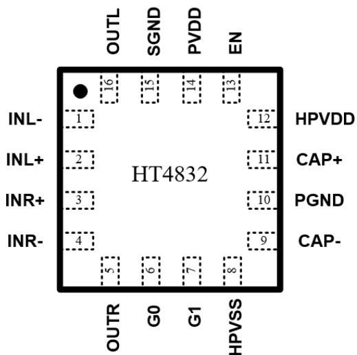
QFN16 顶视图
