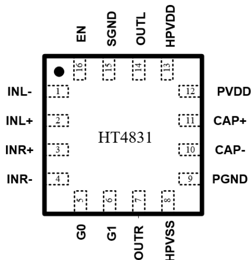
QFN16 顶视图
