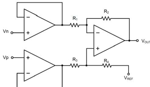
图 5，高输入阻抗差分放大器
