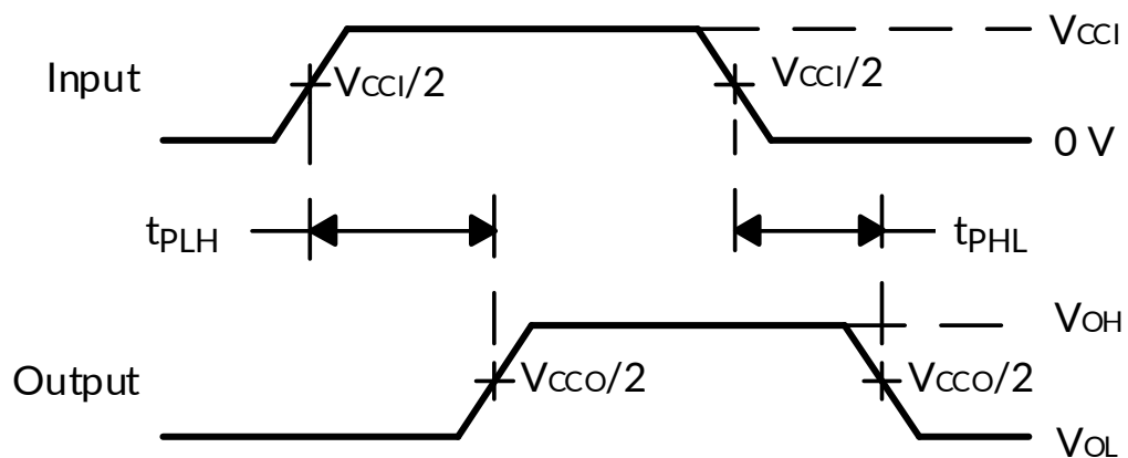
图 2. 电压波形传播延迟时间
