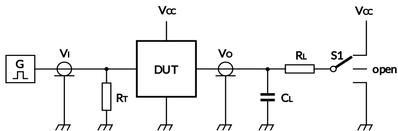
负载电路
