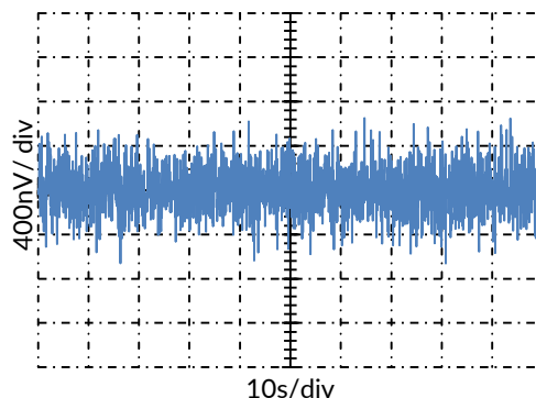
图 16. 0.01Hz ~ 10Hz 输入电压噪声, V_S = 2.7\text{V}
