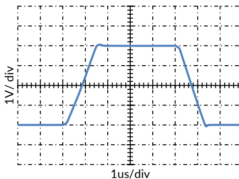
图 12. 大信号阶跃响应, C_L = 100\text{ pF}
