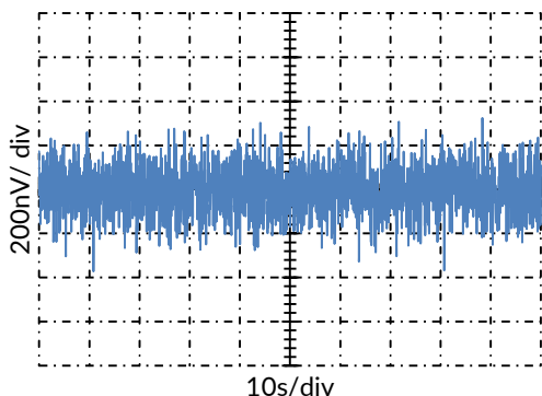
图 15. 0.01Hz ~ 10Hz 输入电压噪声, V_S = 5\text{V}
