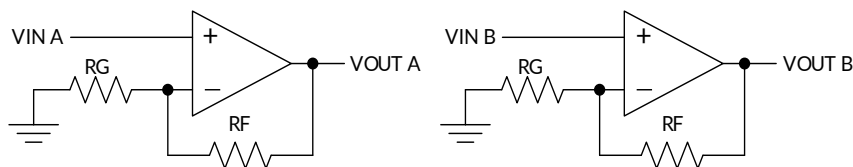
图 21. 应用原理图示意
