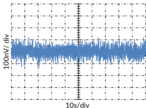
图 17. 0.01Hz ~ 1Hz 输入电压噪声, V_S = 5\text{V}
