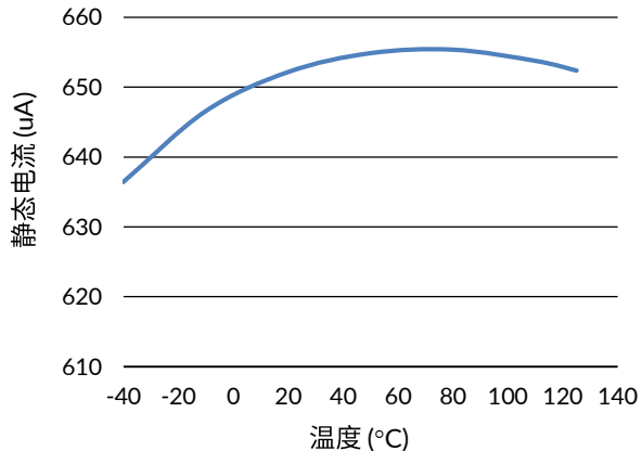
图 8. 静态电流与温度的关系, V_S = 2.7\text{V}
