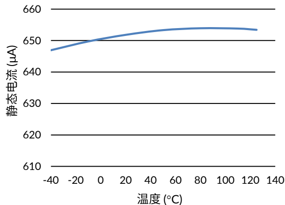
图 7. 静态电流与温度的关系, V_S = 5\text{V}
