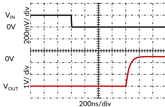
图 14. 反向过载恢复, V_S = \pm 2.5\text{V} , G = -100
