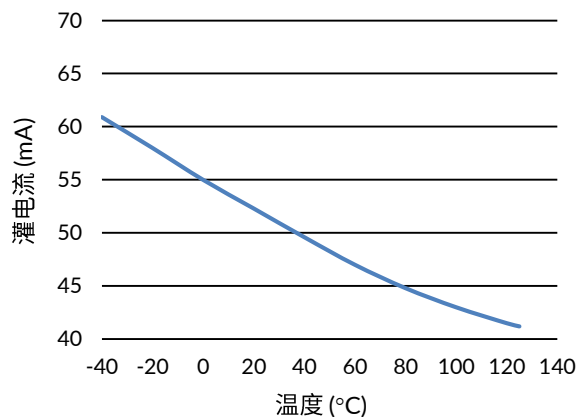
图 10. 灌电流与温度的关系
