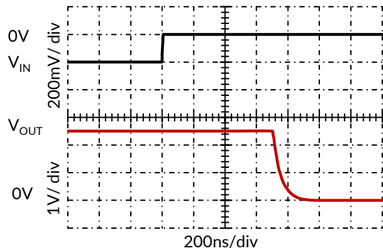
图 13. 正向过载恢复, V_S = \pm 2.5\text{V} , G = -100
