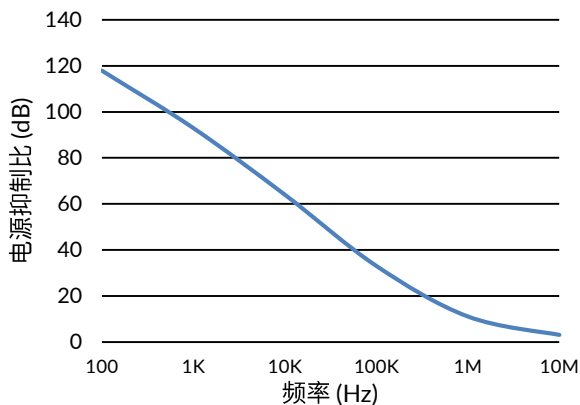
图 5. 电源抑制比与频率的关系
