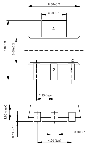
SOT-223
