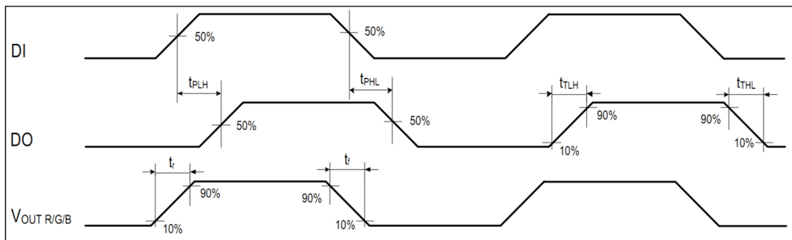
动态参数测试示意图
